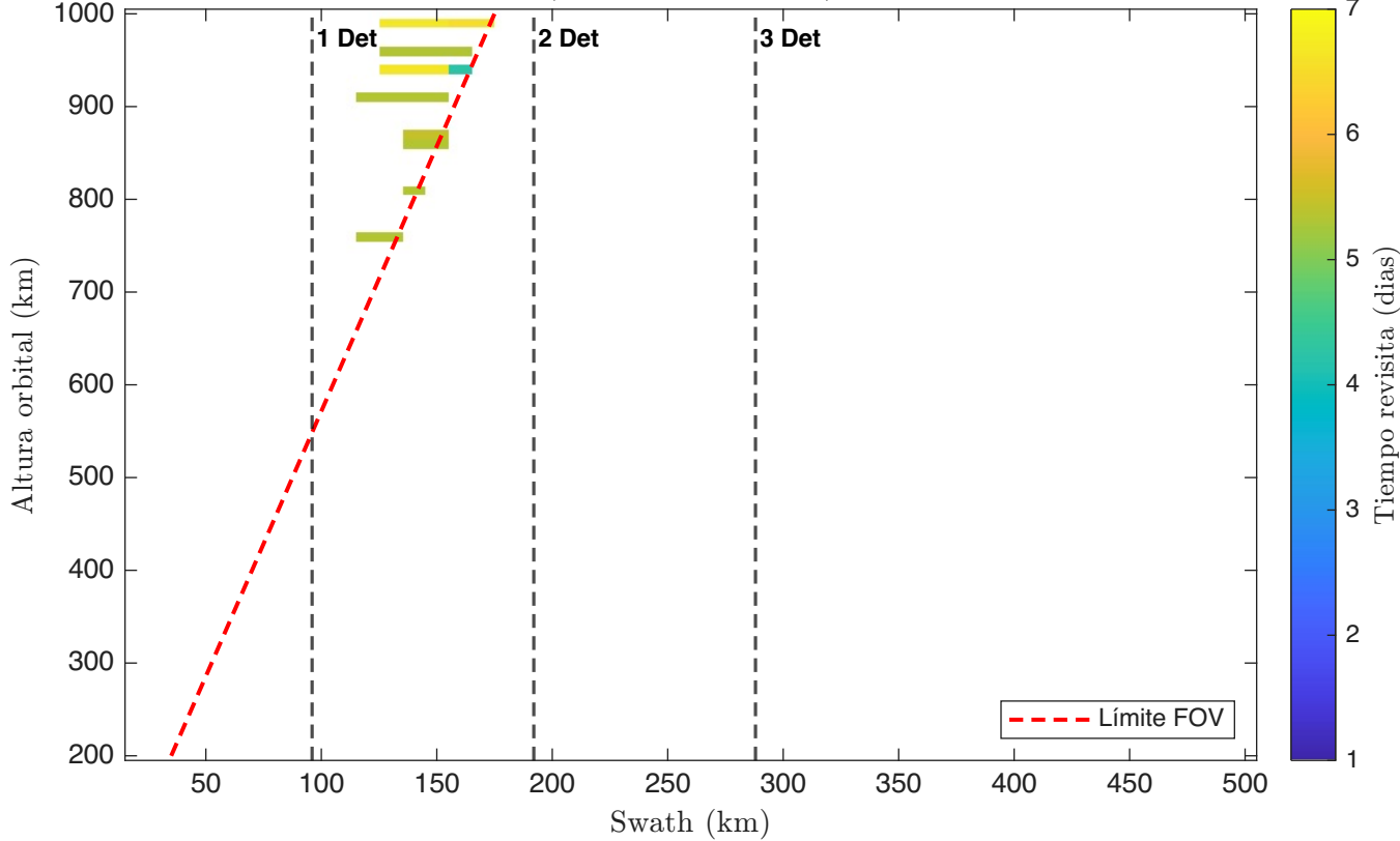
Tiempo Revisita - 3 Satelite(s); 1 Telescopio(s): Refractivo; Detector 1 (Blanco: \geq 7 dias)
